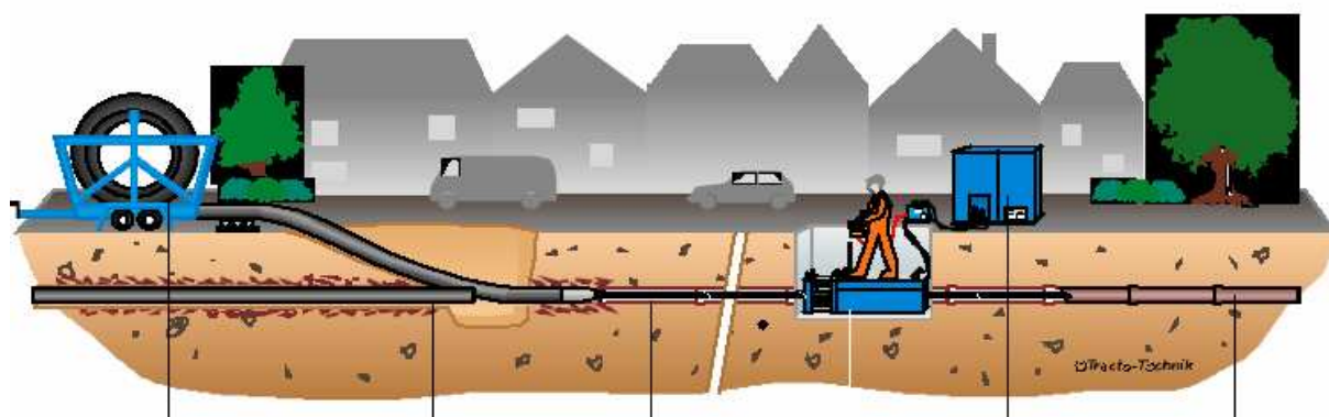
naviják trubky
